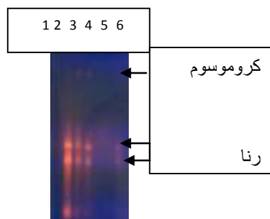
شكل(5). الترحيل الكهربائي لمستخلصات دنا بكتريا B. stearothermophilus المعاملة بالرصاص باستخدام هلام الاكاروز بتركيز 1% و 5 فولت/ سم. (1- نموذج السيطرة ، 2- تركيز 0.2 ملي مولاري رصاص ، 3- تركيز 2مليمولاري رصاص ، 4- نموذج 4 ملي مولاري رصاص)
