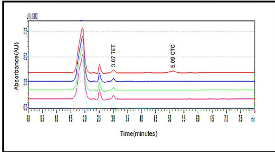
شكل (6) رسم كروماتوجرافي يوضح بعض العينات التي تحتوي على بقايا التتراسيكلين والكلورتتراسيكلين
