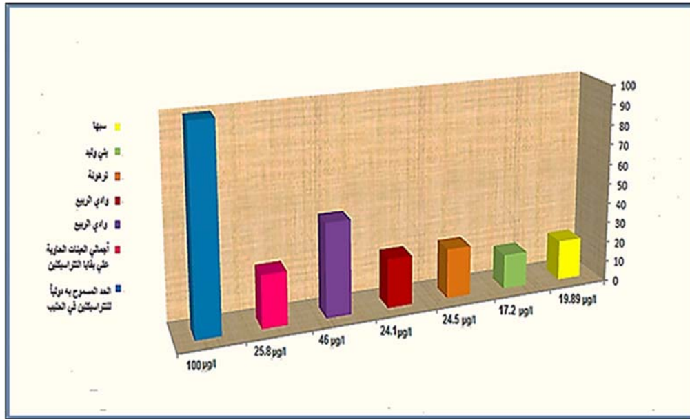
شكل (7). تركيز بقايا التتراسيكلين (ppb) في (50) عينة حليب والحد المسموح به في الحليب.
