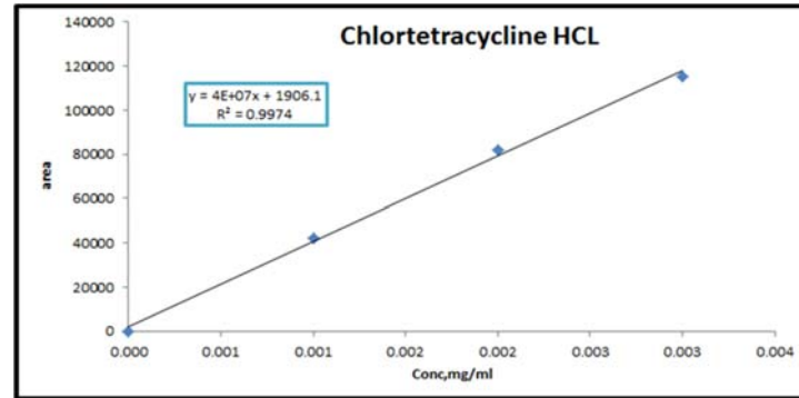
شكل (4) منحنى المعايرة للكلور تتراسيكلين.
