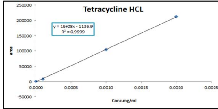
شكل (2) منحنى المعايرة للتتراسيكلين.
