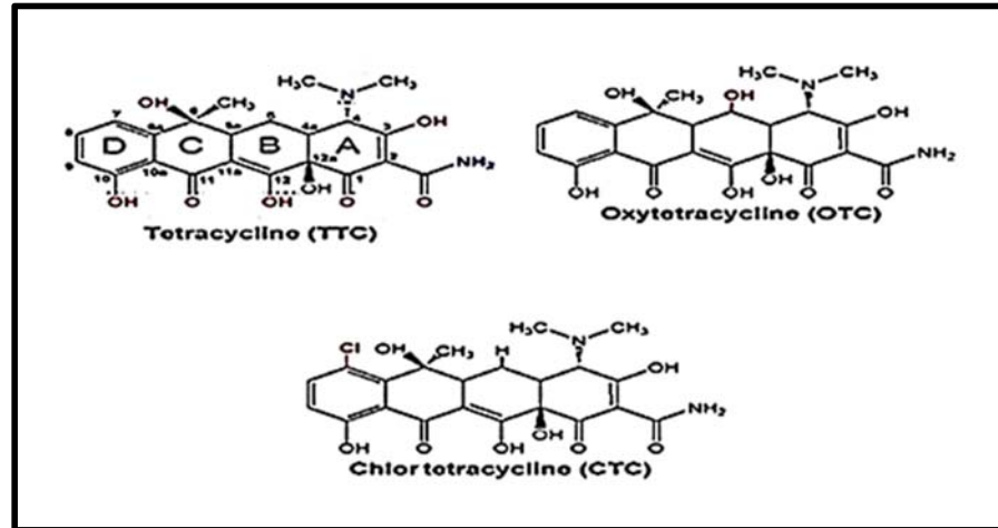
شكل (1). التركيب الكيميائي للمضاد الحيوي التتراسيكلين، الأوكسي تتراسيكلين، الكلور تتراسيكلين
