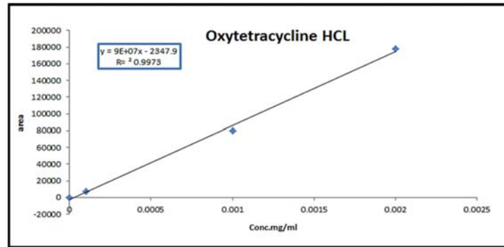
شكل (3) منحنى المعايرة للأوكسي تتراسيكلين.
